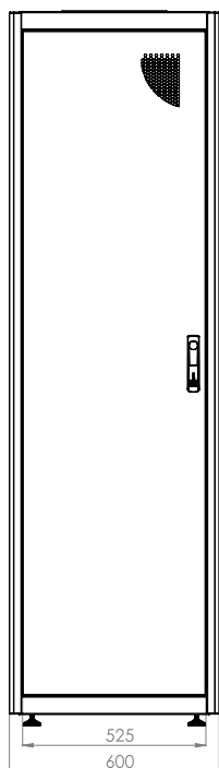
ВИД СПЕРЕДИ
