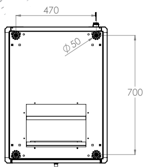
ВИД СНИЗУ
