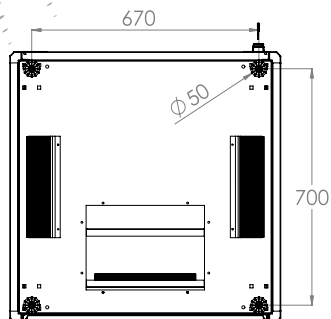
ВИД СНИЗУ
