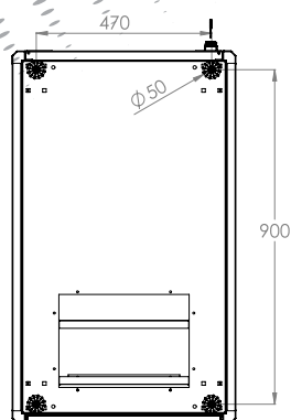
ВИД СНИЗУ
