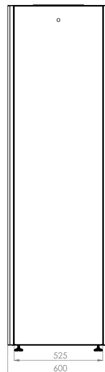
ВИД СЗАДИ
