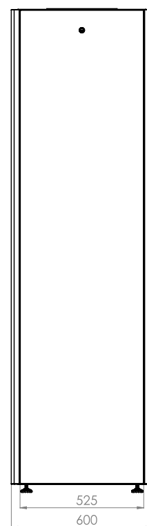
ВИД СЗАДИ
