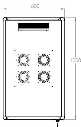
ВИД СВЕРХУ
