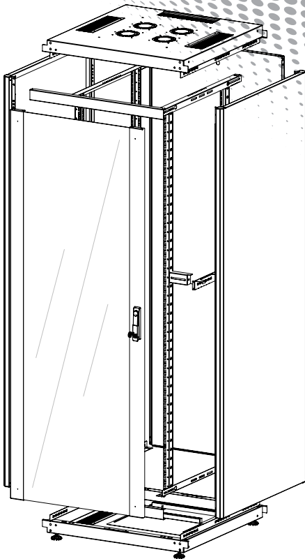
ДЕТАЛЬНЫЙ ВИД
