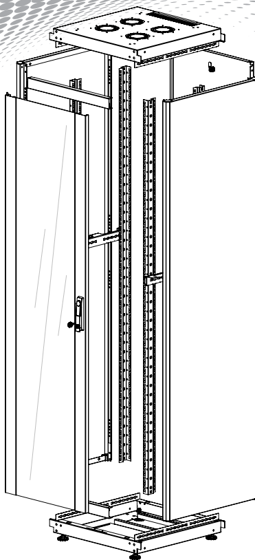
ДЕТАЛЬНЫЙ ВИД
