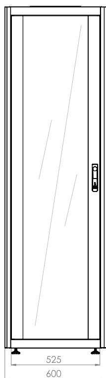
ВИД СПЕРЕДИ
