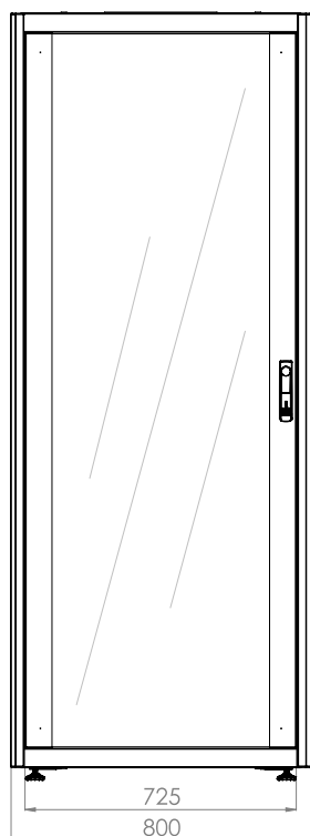
ВИД СПЕРЕДИ
