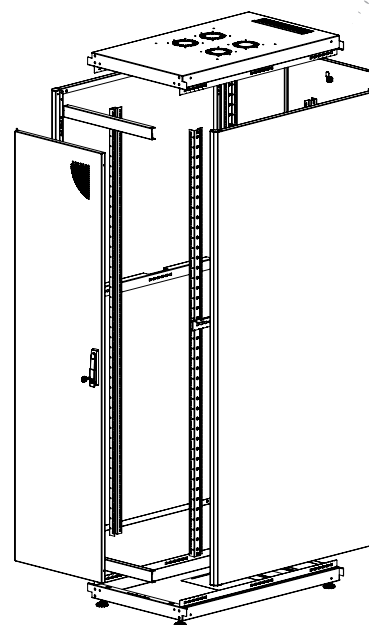
ДЕТАЛЬНЫЙ ВИД
