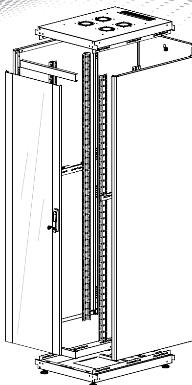
ДЕТАЛЬНЫЙ ВИД
