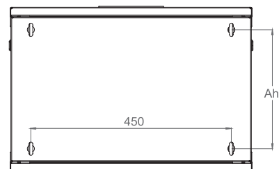
Вид сзади
