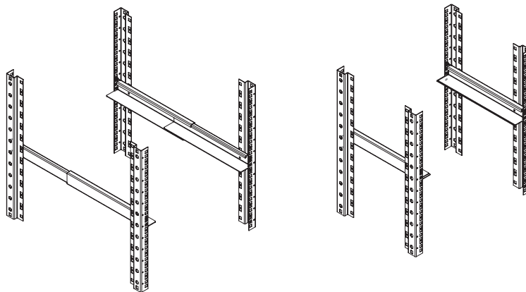
ДИАПАЗОН МОНТАЖА
