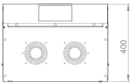
Вид сверху
