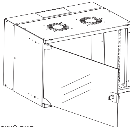
Изометрический вид
