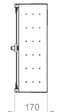
Вид справа
