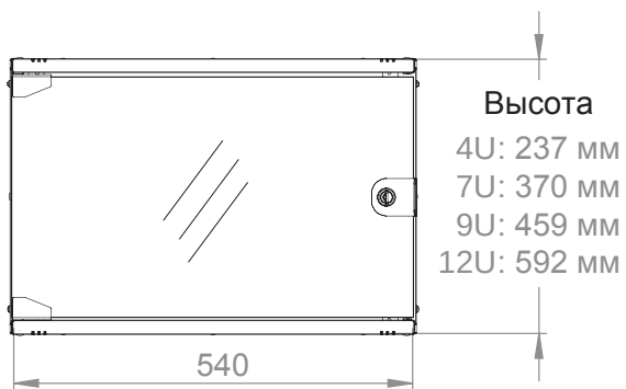
Вид спереди
