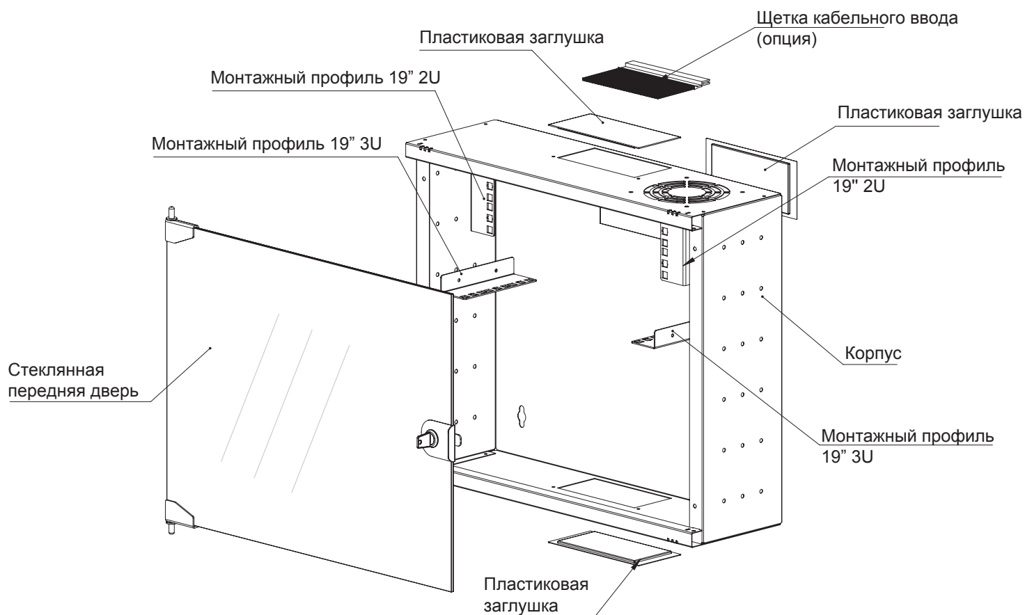
19" SET SLIM Настенный шкаф Ш=540 мм Г=170 мм
