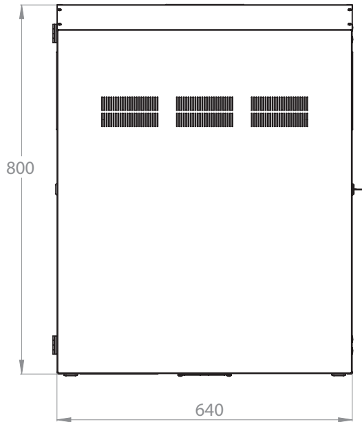
ВИД СПЕРЕДИ
