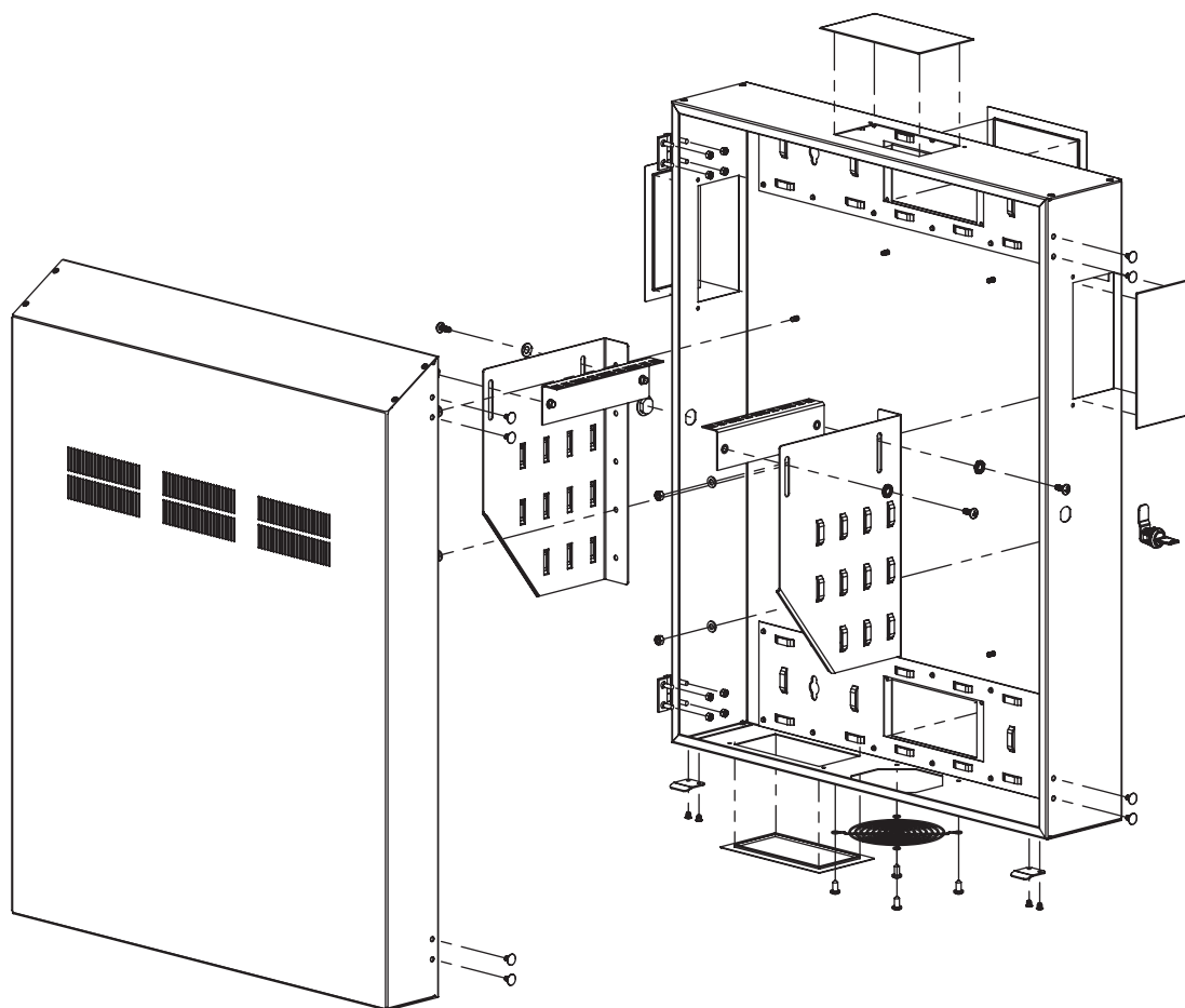
ДЕТАЛЬНЫЙ ВИД
