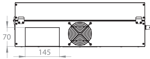
ВИД СНИЗУ
